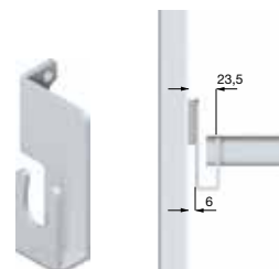
O3012 držák šatní tyče - pár
