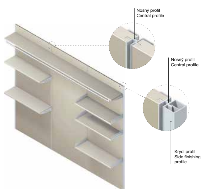
Použití systému CLICK včetně panelů
