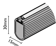
O3622 šatní tyč s těsněním
