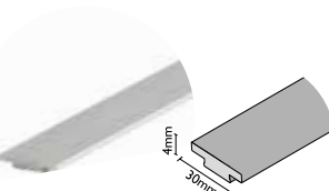
O3602 krycí profil plochý hladký
