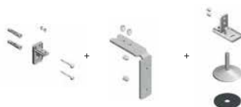
O3002 sada kování pro uchycení podlaha / stěna
