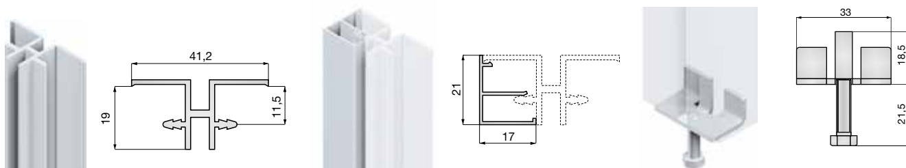
O3200 nosný profil 2650 mm
