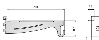
O3209 podpora s držákem šatní tyče
