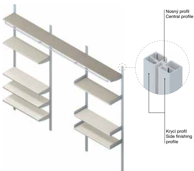
Použití systému CLICK bez panelů
