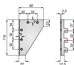
O3212 úchyt na skříňku
