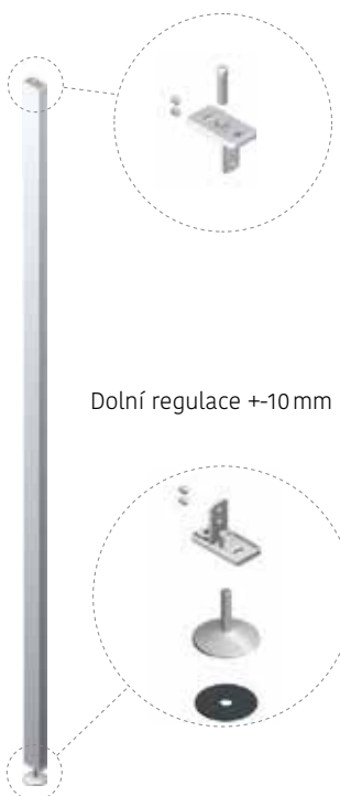
Sestava "I" - podlaha/strop
