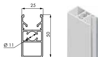
O3000 nosný profil 3050 mm
