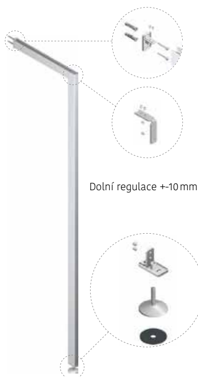
Sestava "L" - podlaha/zed'
